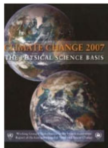
AR4 2007
