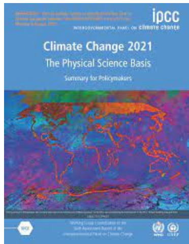
AR6 2021-2023
